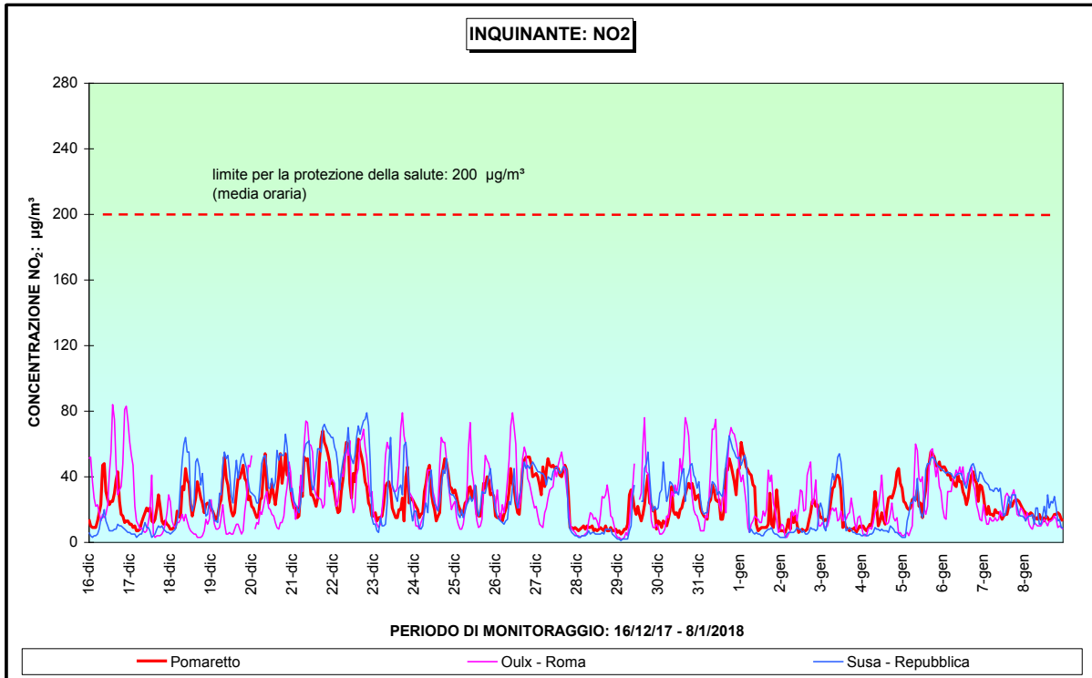
Figura 17 – NO 2 : confronto con i dati di altre stazioni di monitoraggio
